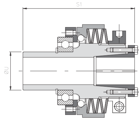
.../P/ML (versione con mozzo lungo)
