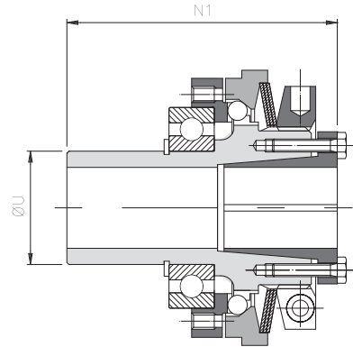
.../N/ML (versione con mozzo lungo)
