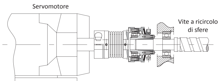
Modello DSS/SG/N montato con giunto a soffietto GSF tra servomotore e vite a ricircolo di sfere
