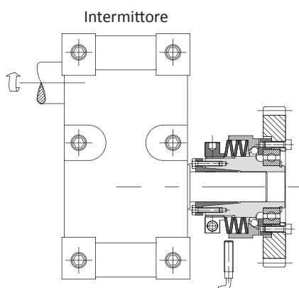
Modello DSS/F/SG/P montato in uscita ad un intermittente
