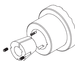
Tipo G Bloccaggio con Taper-bush interno.
