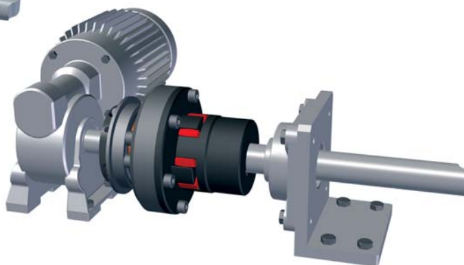
Trasmissione ad alberi coassiali
