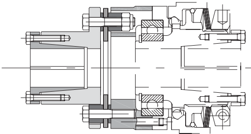
Modello DSS/SG/RF con giunto torsionalmente rigido a lamelle singolo GTR/S , per applicazioni dove sia richiesta rigidità e assenza di gioco torsionale.
