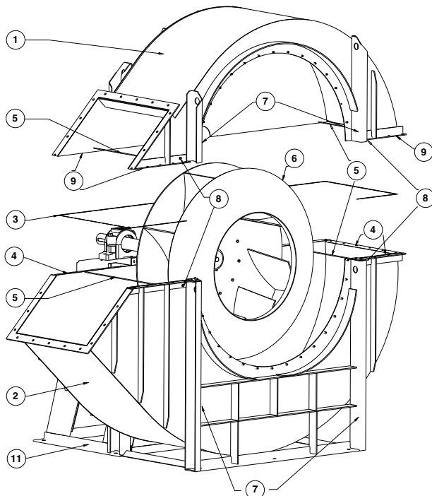
disegno 1 / drawing 1 / dessin 1 / Zeichnung 1 / plano 1 / desenho 1
