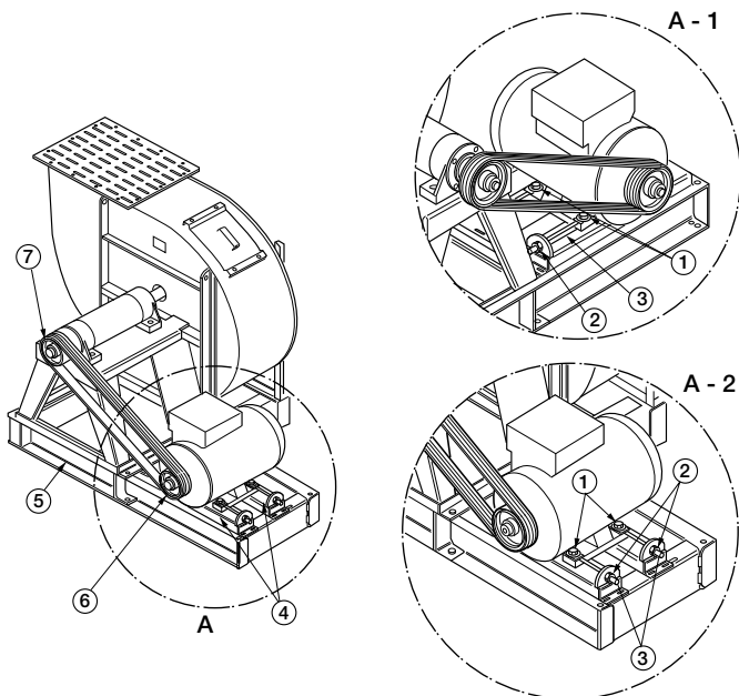
disegno 2 / drawing 2 / dessin 2 / Zeichnung 2 / plano 2 / desenho 2
